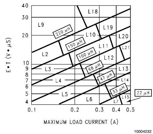
FIGURE 7. LM2671-ADJ
